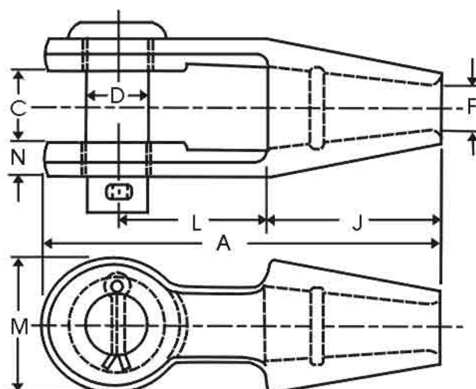
OPEN SPELTER SOCKETS
